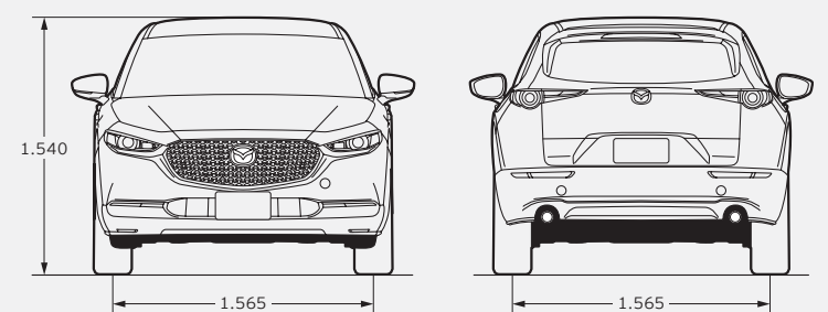
DIMENSIONES Unidad: mm
